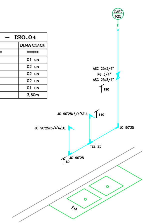
ISOMÉTRICO 04 ESC:..1/25
